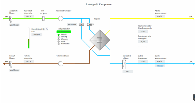
Integration eines Lüftungsgeräts im Klassenraum. Integration of a ventilation unit in the classroom.
